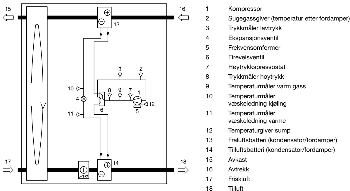
Flytskjema for kjølemiddelsystem
