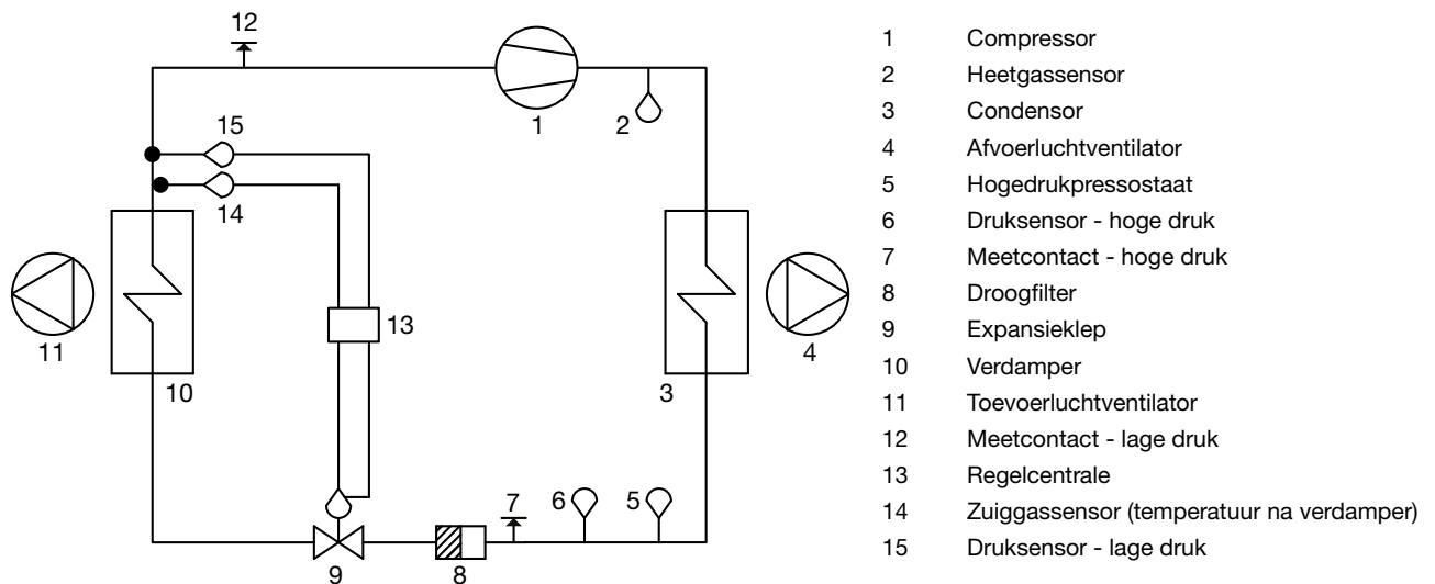
Stroomschema voor koelmiddelsysteem grootte 04-12
