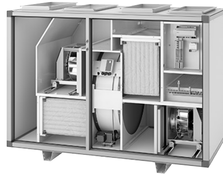
Envistar Top met roterende warmtewisselaar (code TEM)
