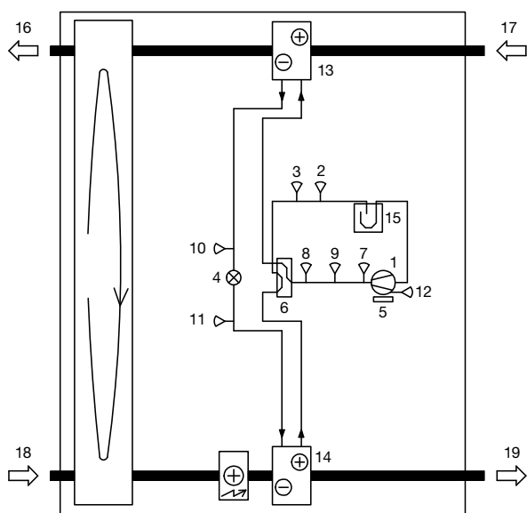
Stroomschema voor koelingsmodus koelwarmtepomp
