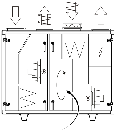
Warmtewisselaarrotor
