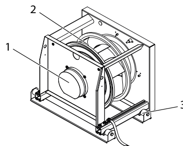
Ventilatorenhed størrelse 10 og 16
