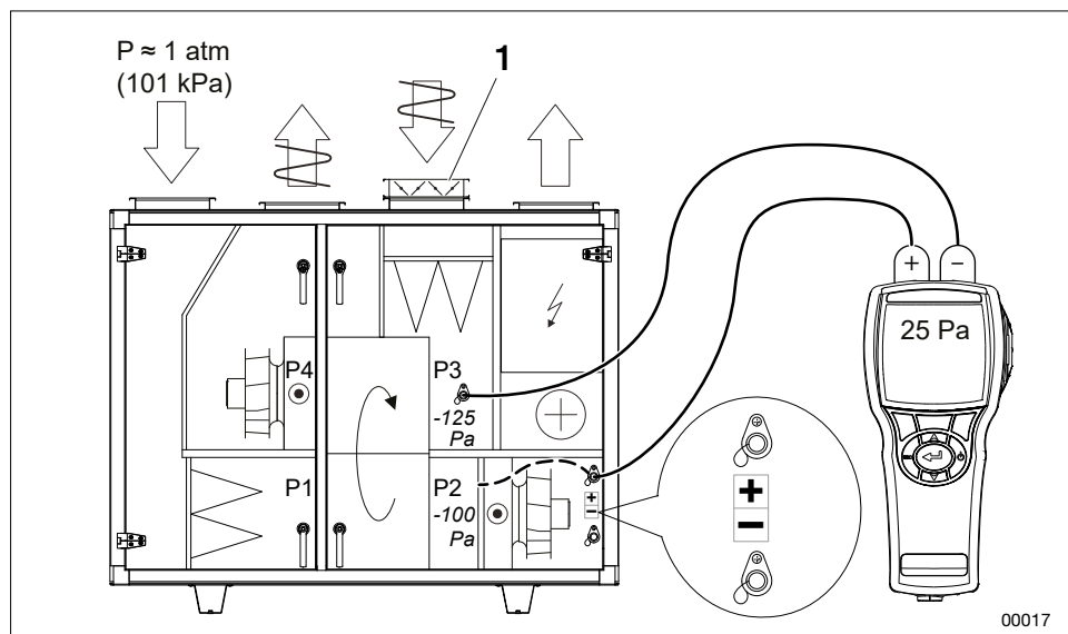
Painetasapainon mittausliitäntä – ilmastointikone ilman ohjauslaitteistoa (koodi UC, MK, US)
