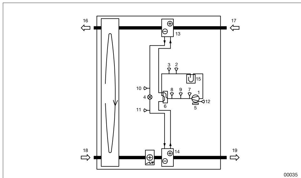
Flödesschema för kyläge kylvärmepump
