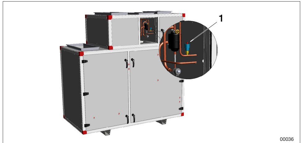
1. Återställningsknapp pressostat
