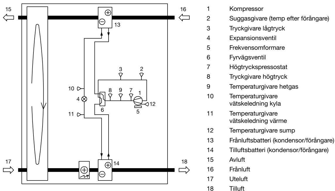
Flödesschema för köldmediesystem
