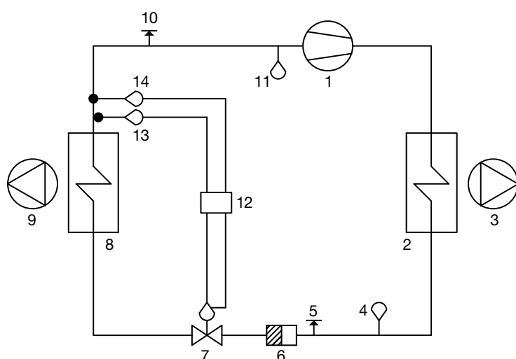
Flödesschema för köldmediesystem storlek 16-21
