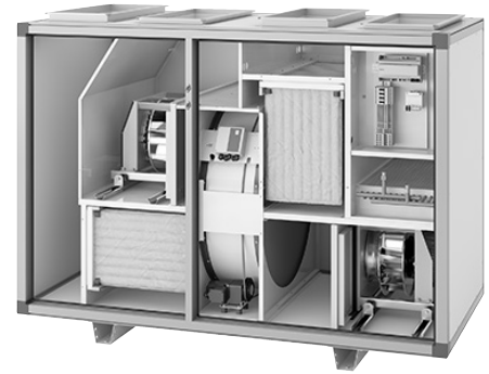
Envistar Top med roterande värmeväxlare (kod TER)
