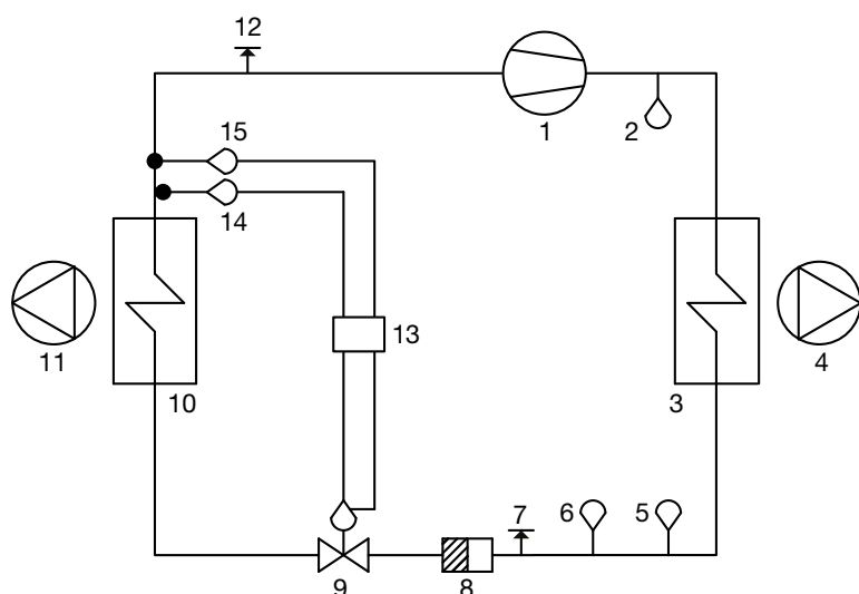
Flödesschema för köldmediesystem storlek 04-12
