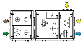
Mit Kältemaschine, Zuluft nach unten
