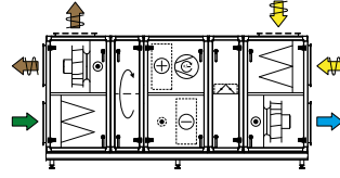
Kombi 5 Rotor, Kältemaschine und Umluftteil
