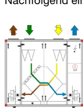
Einheitl. Ausführung Größe 04, 06 und 10
