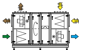
Kombi 4 Rotor und Umluftteil
