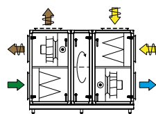
Kombi 1 Rotor
