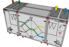
Größe 09, 10, 12, 17, 22 und 28, geteilter Gegenstromwärmetauscher
