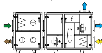
Mit Kältemaschine, Zuluft nach oben
