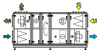
Kombi 3 Kältemaschine mit Kälterückgewinnung
