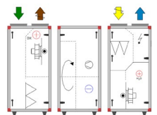
Größen 09, 12, 17 i und 22 i mit Kältemaschine
