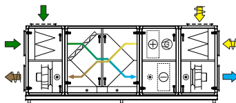
Kombi 8 Gegenstromwärmetauscher und Kältemaschine
