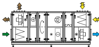
Kombi 6 Kältemaschine mit Kälterückgewinnung und Umluftteil
