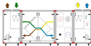
Größe 09, 10, 12, 17, 22 und 28 mit integrierter Kältemaschine
