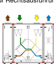
Geteilte Ausführung Größe 04, 06 und 10
