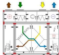
Geteilte oder Blockausführung in den Größen 04, 06 und 10 mit integrierter Kältemaschine
