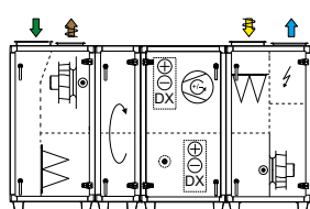
Rotor und Reversible Wärmepumpe Größen 09, 12, 17 und 22
