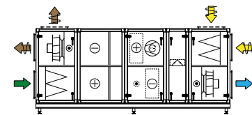
Kombi 14 Kreislaufverbundsystemteil, Kältem., Umluftteil
