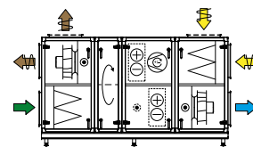
Rotor und Kühl-/Wärmepumpe
