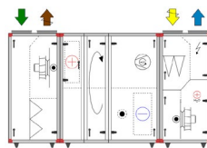
Größe 17 h , 22 h und 28 mit Kältemaschine
