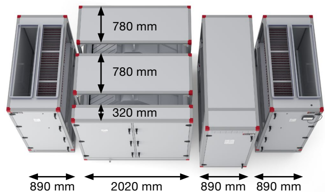
Envistar Top Größe 28 mit EcoCooler und geteiltem Gegenstromwärmetauscher.
