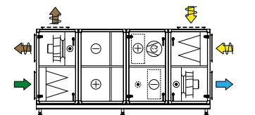
Kombi 12 Kreislaufverbundsystemteil und Kältemaschine
