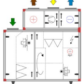
Größen 04, 06 und 10 mit Kältemaschine
