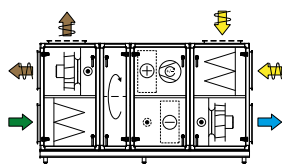
Kombi 2 Rotor und Kältemaschine
