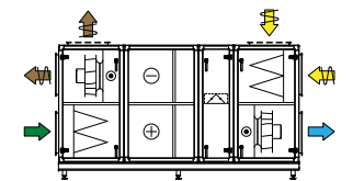
Kombi 13 Kreislaufverbundsystemteil und Umluftteil
