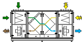
Kombi 7 Gegenstromwärmetauscher
