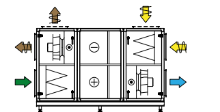
Kombi 11 Kreislaufverbundsystemteil
