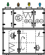
Rotor und Reversible Wärmepumpe Größen 06 und 10
