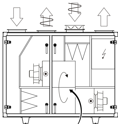
Återvinnare rotor
