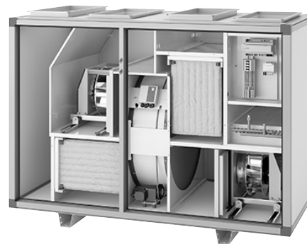
Envistar Top med roterande värmeväxlare (kod ATER)
