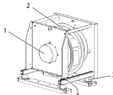
Fläktenhet storlek 10-21
