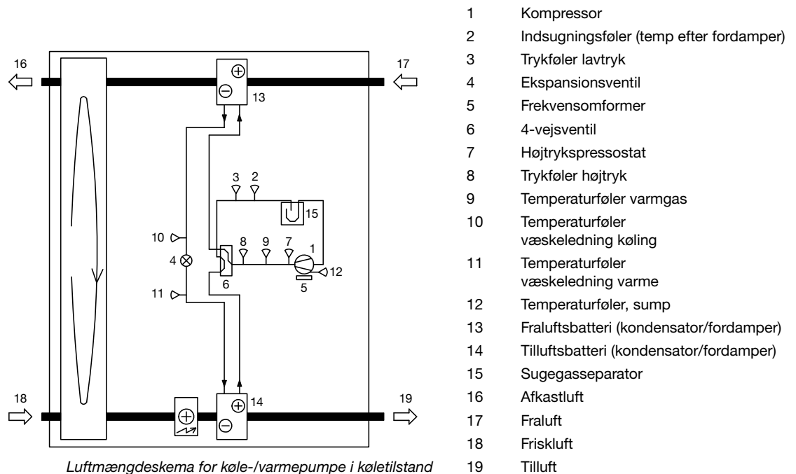
Luftmængdeskema for køle-/varmepumpe i køletilstand
