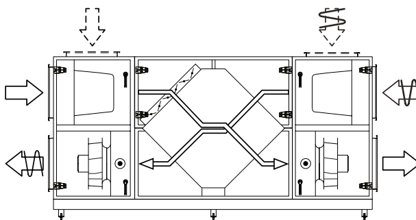
Plattvärmewäxlare av typen motström, EXM
