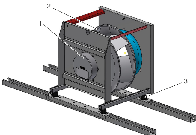
Exempel på fläkt storlek 240–980
