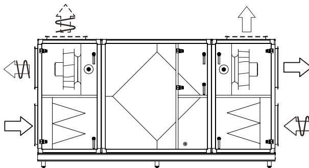
Plattvärmewäxlare av typen korsström, EXP
