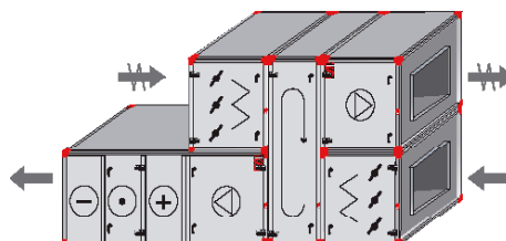
Till- och frånluftsaggregat, 2-höjd
