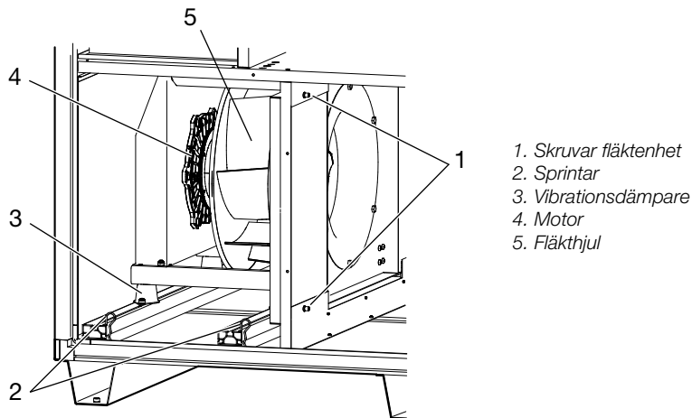
Fläktenhet storlek 10 och 16
