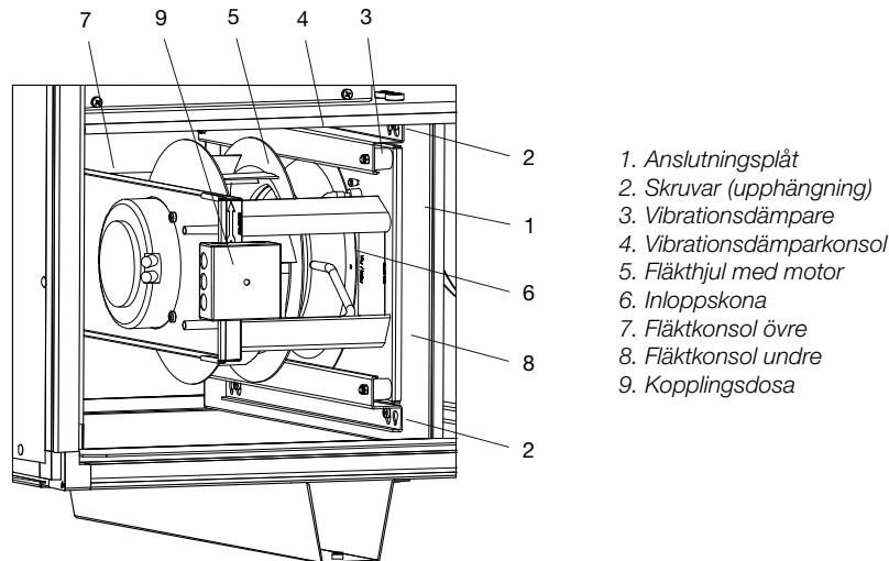
Fläktenhet storlek 04 och 06
