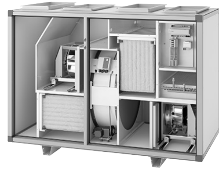
Envistar Top med roterende varmeveksler (kode TER)
