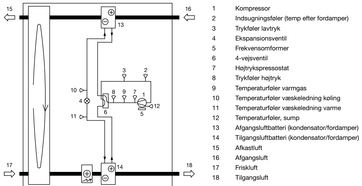
Strømningskema for kølemiddelsystem
