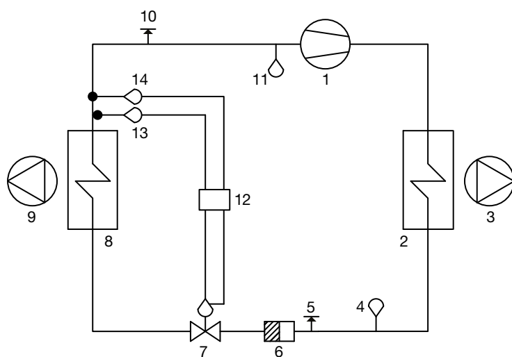
Strømningsskema for kølemiddelsystem, størrelse 16-21
