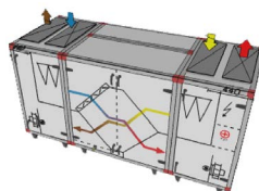
Størrelse 09, 10, 12, 17, 22 og 28, delt motstrømsveksler
