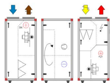
Størrelse 09, 12, 17 og 22 med integrert kjøling
