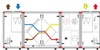
Størrelse 09, 10, 12, 17, 22 og 28 med med integrert kjøling
