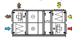
Komb. 13 Batterigjennvinningsdel og omluftsdel
