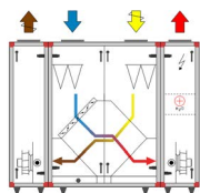
Delt utførelse størrelse 04, 06 og 10
