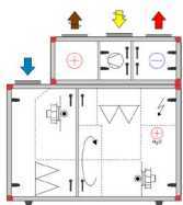
Størrelse 04, 06 og 10 med integrert kjøling
