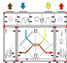
Delat- eller enhetsutførende størlek 04, 06 och 10 med med integrert kjøling
