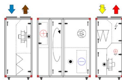
Størrelse 28 med integrert kjøling
