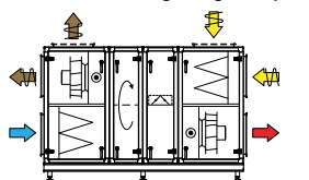
Komb. 4 Rotor og omluftsdel
