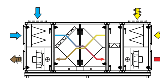
Komb. 9 Motstrømsvarmeveksler og omluftsdel
