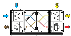
Komb. 7 Motstrømsvarmeveksler
