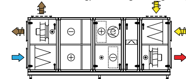
Komb. 14 Batterigjennvinningsdel, integrert kjøling og omluftsdel
