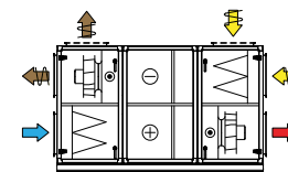
Komb. 11 Batterigjennvinningsdel
