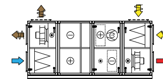
Komb. 12 Batterigjennvinningsdel og integrert kjøling
