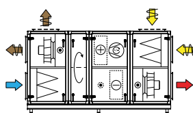
Komb. 2 Rotor og integrert kjøling
