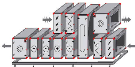
Geteilte Ausführung mit Tragplatte
