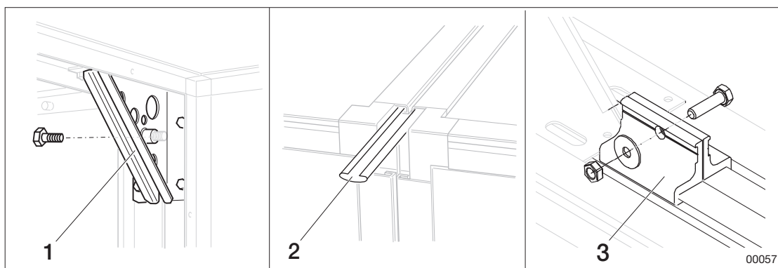
Abbildung: Schraubverbindungen und Klemmlaschen
