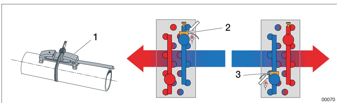
Abbildung: Auflagensensor
