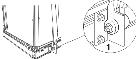
Abbildung: Am Trägerrahmen vormontierte Hebeöse
