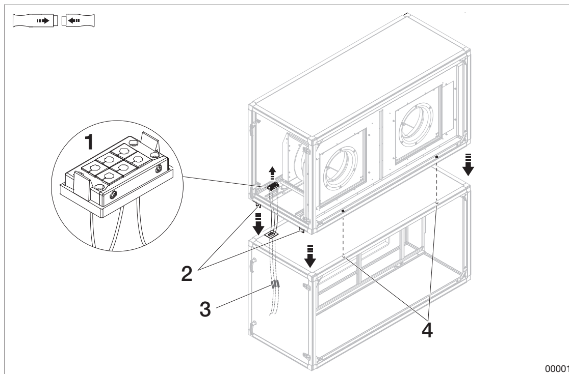
Abbildung: Ventilator- und Filterteil (ENF)
