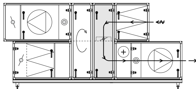
Принципиальная схема – рециркуляция воздуха в секции рециркуляции (отмечена серым цветом).
