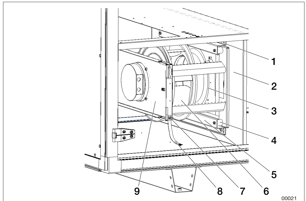
Beispiel Ventilatoreinheit Größe 04–06
