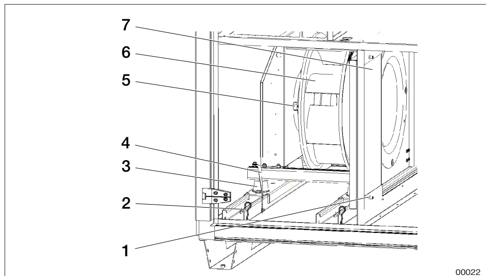
Beispiel Ventilatoreinheit Größe 09-21
