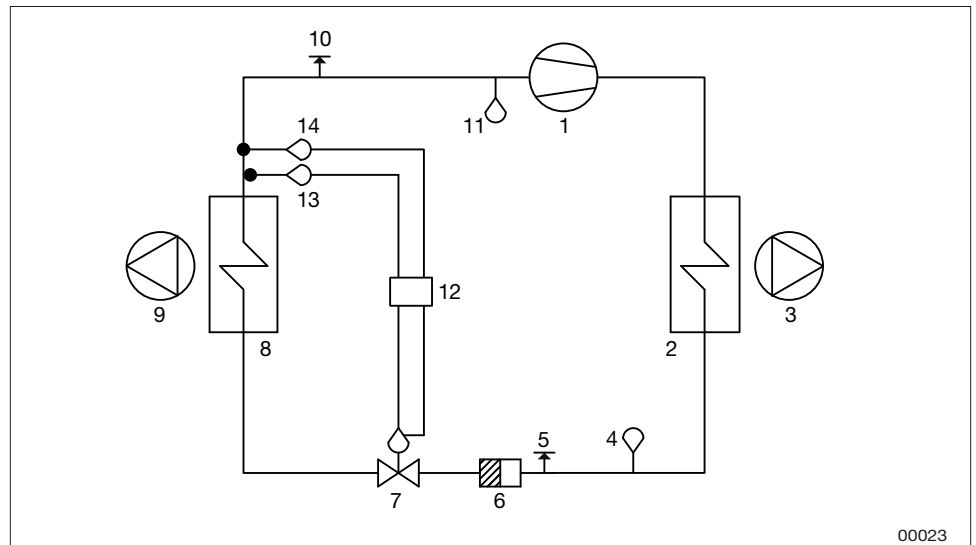
Fließschema für Kältemittelsystem Größe 16–21
