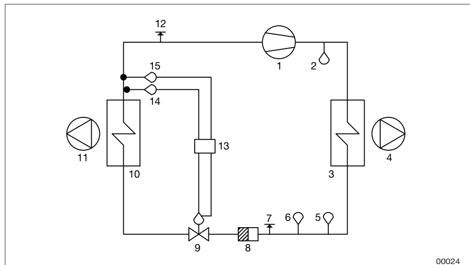
Fließschema für Kältemittelsystem Größe 04-12
