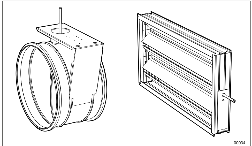
Jalousieklappe ETSP-UM, ETSP-TR und ETSP-UM, ETSP-TR, ETRL
