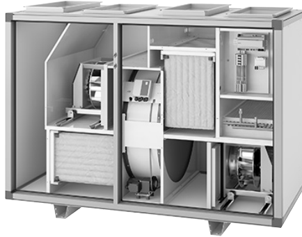
Envistar Top mit rotierendem Wärmetauscher (Code TER)
