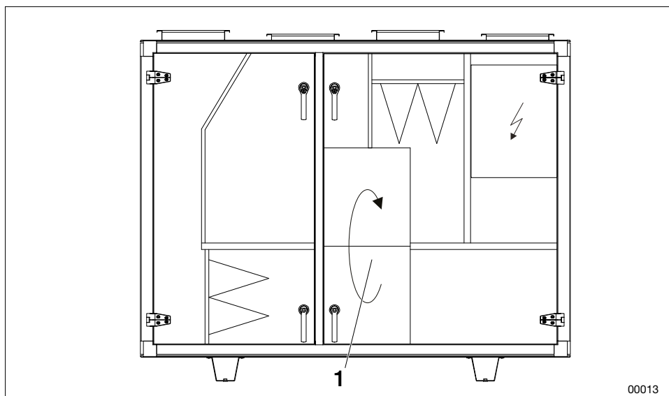
1. Wärmerückgewinnung, Rotor
