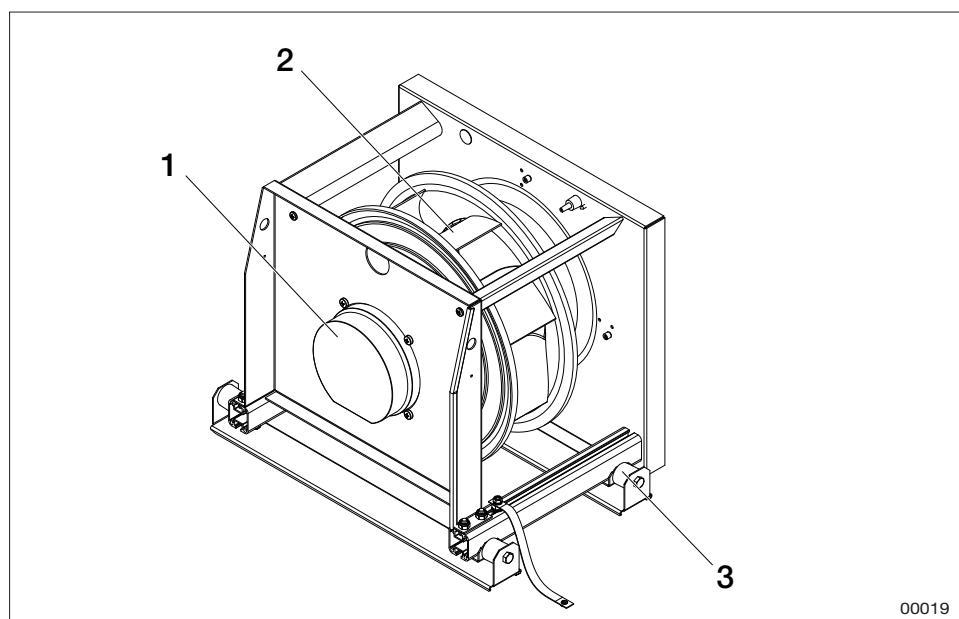
Beispiel Ventilatoreinheit Größe 09-21
