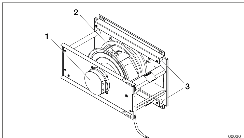
Beispiel Ventilatoreinheit Größe 04-06
