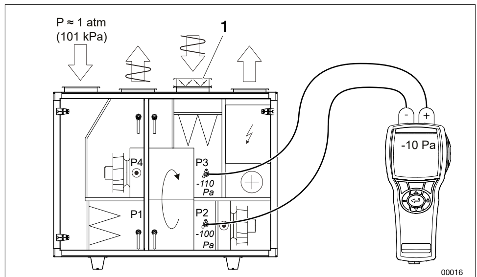
Messanschluss für Druckausgleich - Gerät der Ausführung Home Concept.
