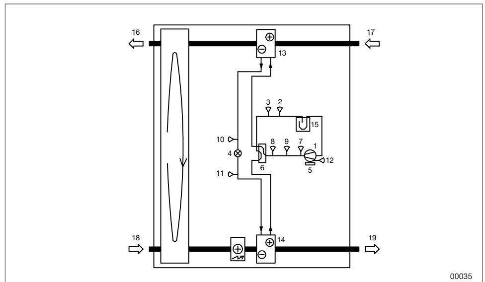
Fließschema für reversible Wärmepumpe im Kühlmodus
