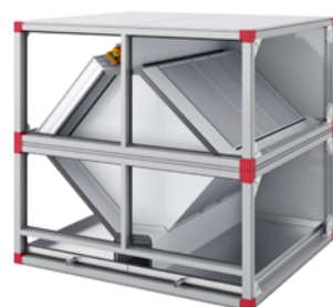
Motströmsväxlare 83 %
