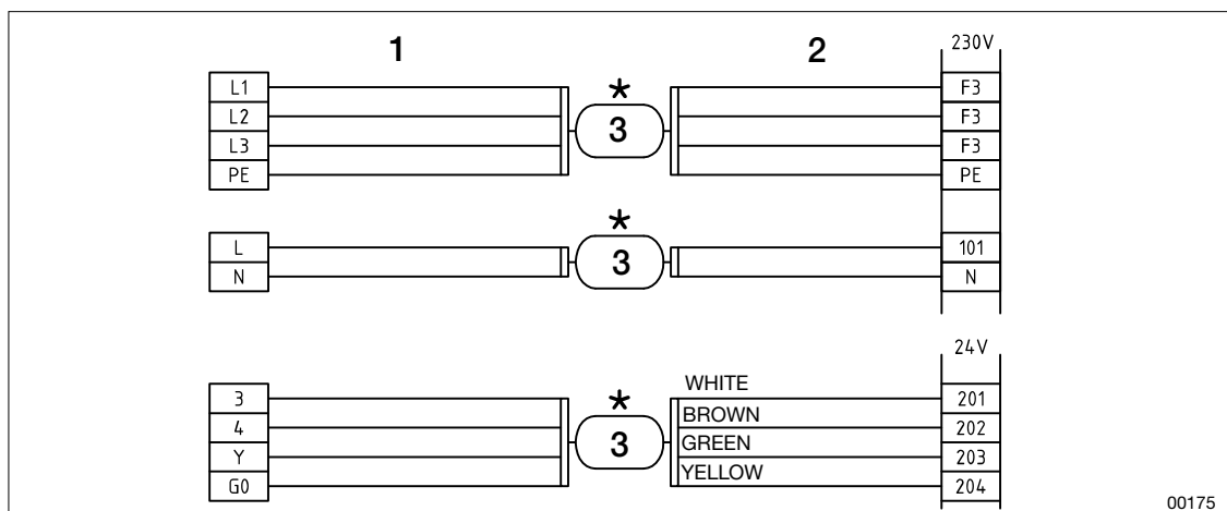
Figur: Inkoppling vid eftermontering
