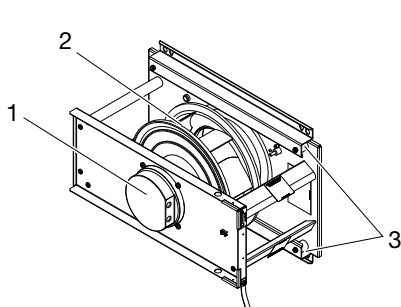
Eksempel på ventilatorenhed størrelse 04-06
