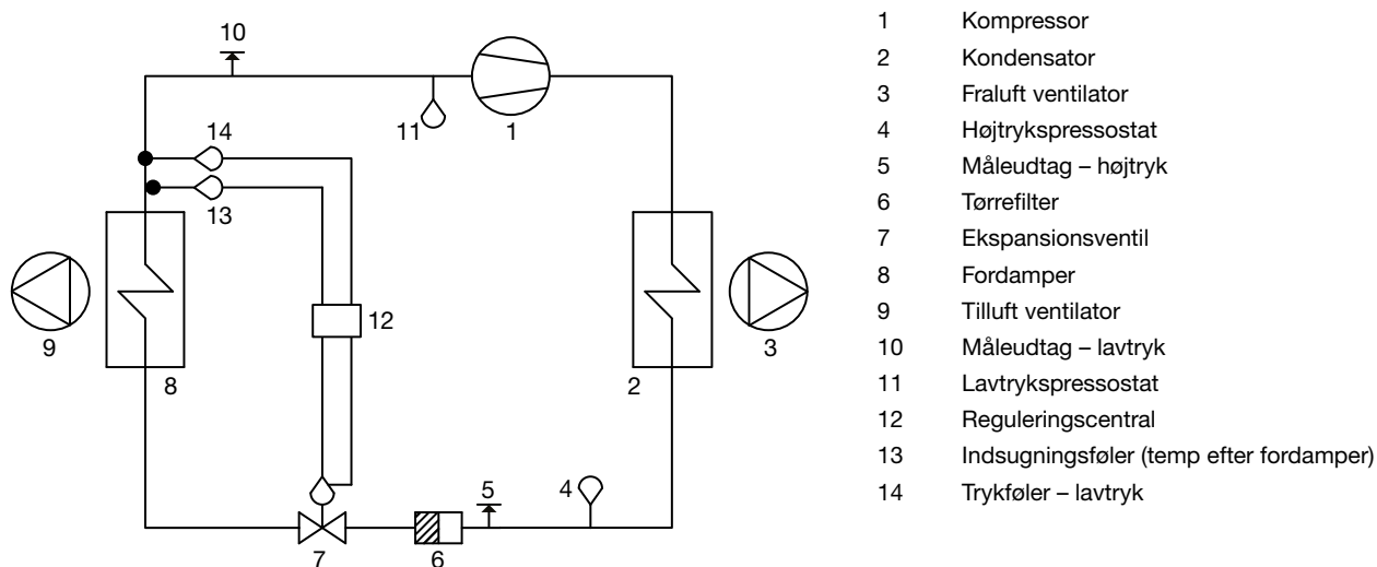
Strømningsskema for kølemiddelsystem, størrelse 16-21
