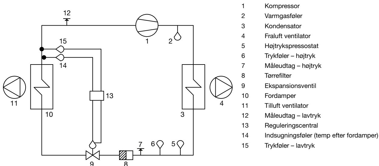
Strømningsskema for kølemiddelsystem, størrelse 04-12
