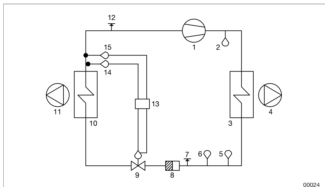
Luftmængdeskema for kølemiddelsystem, størrelse 04-12
