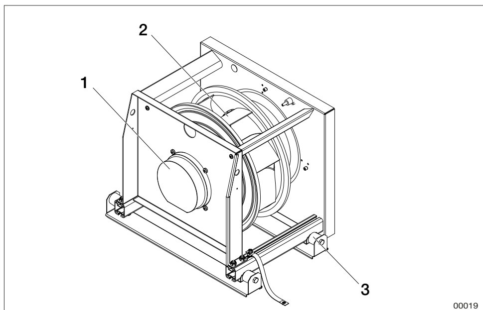
Eksempel på ventilatorenhed størrelse 09-28
