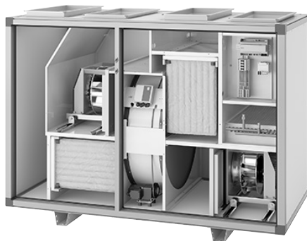
Eksempel på Envistar Top med roterende varmeveksler
