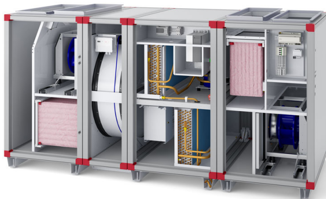
Eksempel på Envistar Top med ThermoCooler HP størrelse 10
