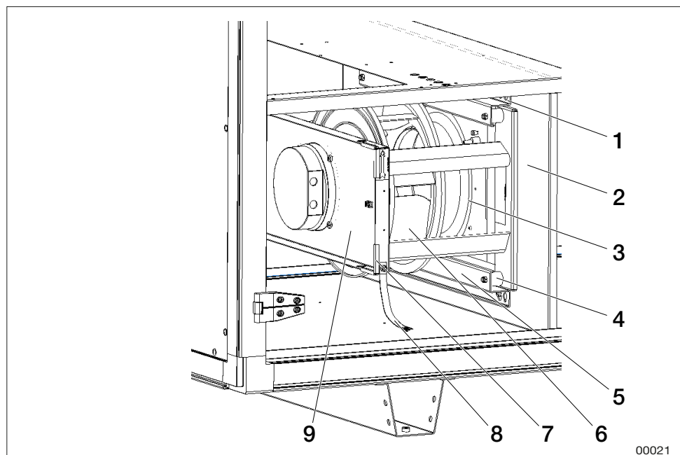
Eksempel på ventilatorenhed størrelse 04-06
