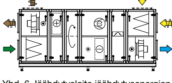
Yhd. 6 Jäähdytyslaite jäähdytysenergian talteenotolla ja sekoitusosa
