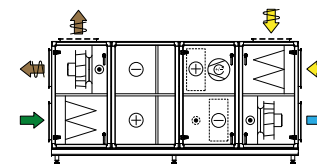
Yhd. 12 Patteritalteenotto-osa ja jäähdytyslaite
