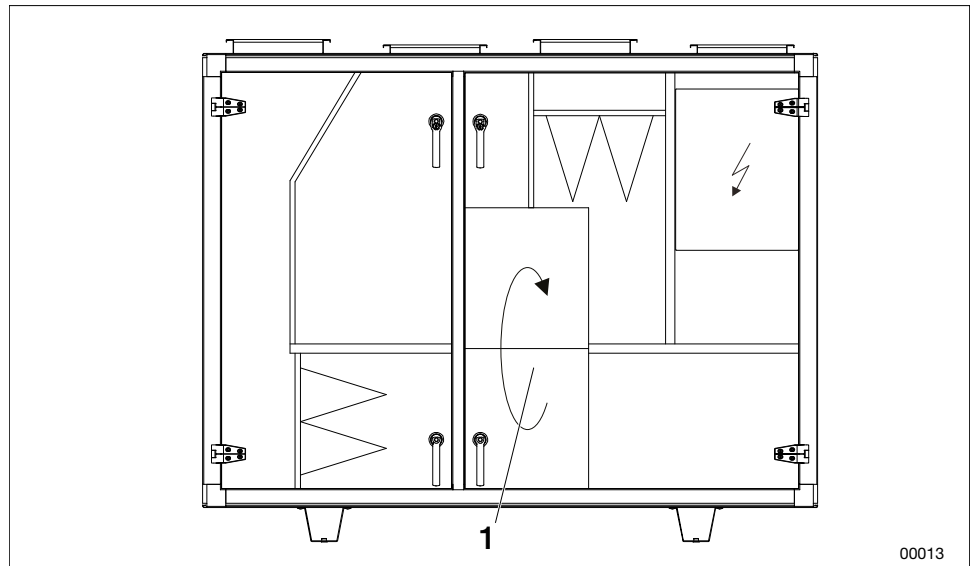
1. Rotor warmtewisselaar
