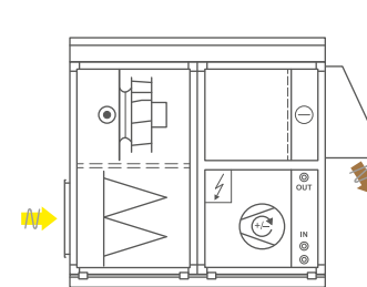
Högerutförande utomhus
