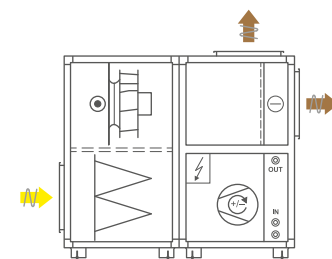
Högerutförande inomhus
