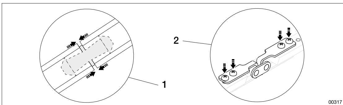
Figur: Tverrsnitt av rundrem og kilerem
