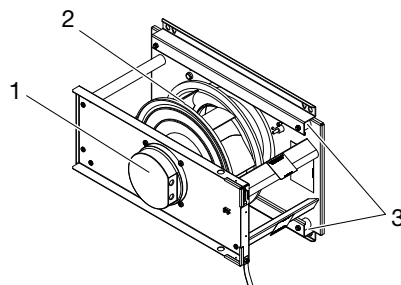
Voorbeeld ventilatoreenheid grootte 04-06
