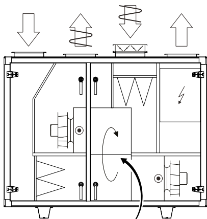
Kierrätysroottori
