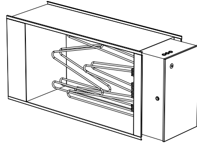
Lämmityspatteri, sähkö koot 04-12 (ETKB-EV)
