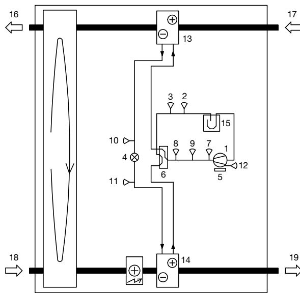
Jäähdytys-/lämpöpumpun jäähdytystilan virtauskaavio
