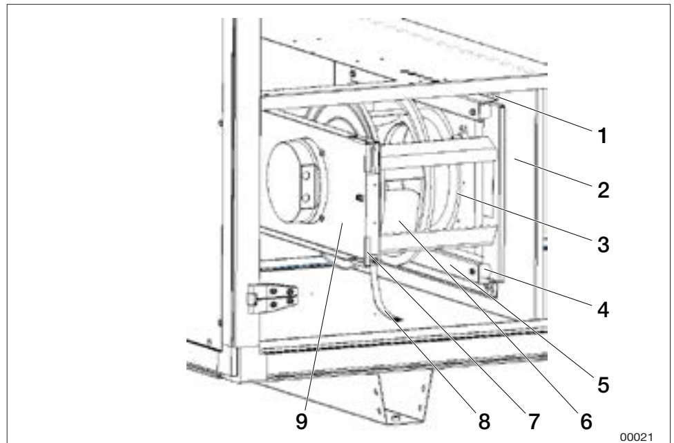
Eksempel på ventilatorenhed størrelse 04-06
