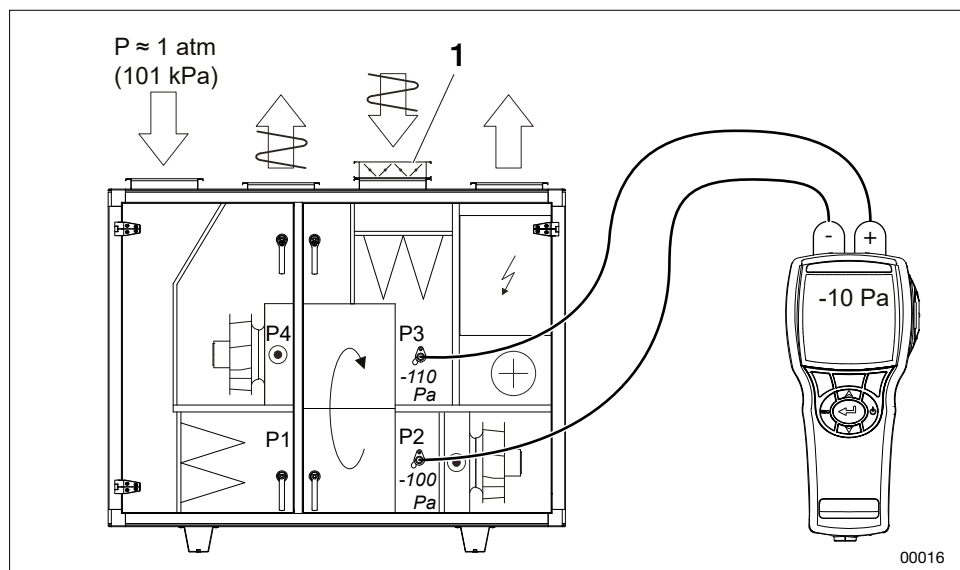
Måleuttak for trykbalanse – aggregat i utførelsen Home Concept.
