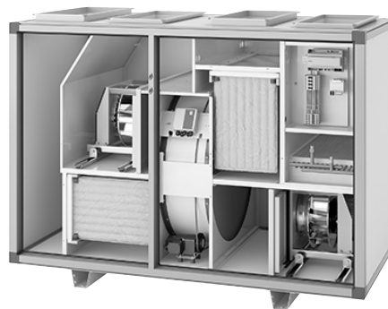
Envistar Top med roterande värmeväxlare (kod TER)
