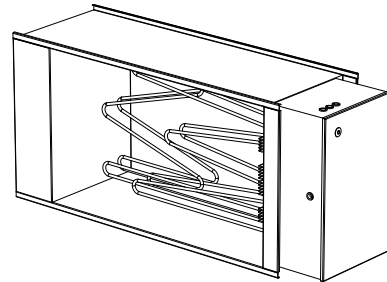
Lufterhitzer Elektro Größe 04-12 (ETKB-EV)
