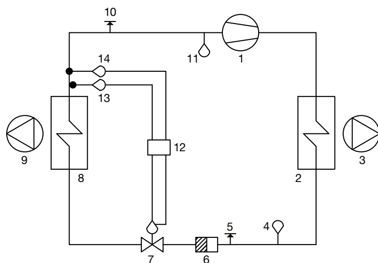
Fließschema für Kältemittelsystem Größe 16-21
