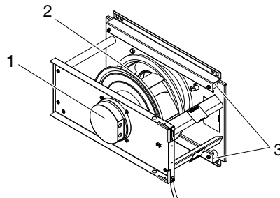
Beispiel Ventilatoreinheit Größe 04-06
