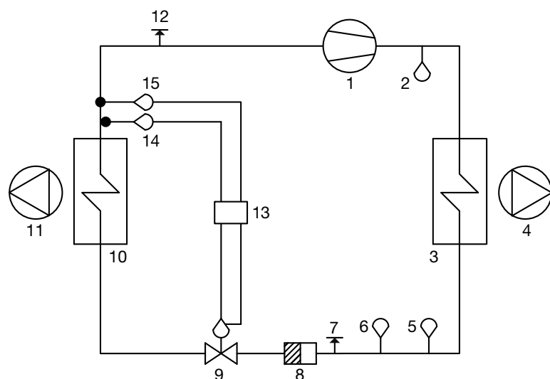
Fließschema für Kältemittelsystem Größe 04-12
