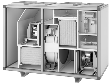
Envistar Top mit rotierendem Wärmetauscher (Code TER)
