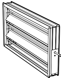
Jalousieklappe Größe 04-21 (ETSP-UM, ETSP-TR, ETRL)
