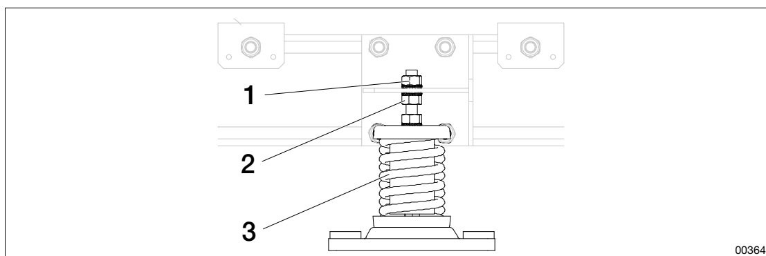
Kuva: Teräsjousivaimennus
