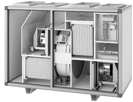
Envistar Top met roterende warmtewisselaar (code TEM)
