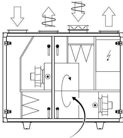
Warmtewisselaarrotor
