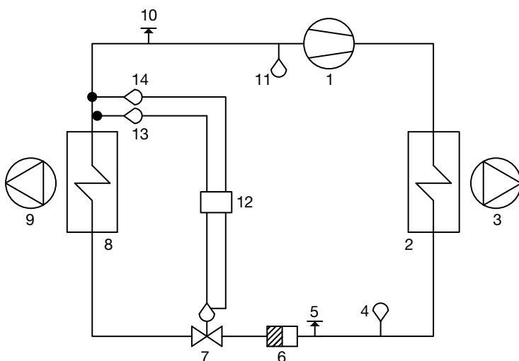
Stroomschema voor koelmiddelsysteem grootte 16-21
