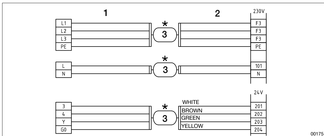
Kuva: ThermoCooler HP:n kytkentä jälkiasennuksessa
