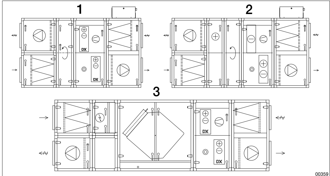
Figur: Eksempler på konfigurationer af ThermoCooler HP. Applikation 3 er tilgængelig på markeder med mildere klima.
