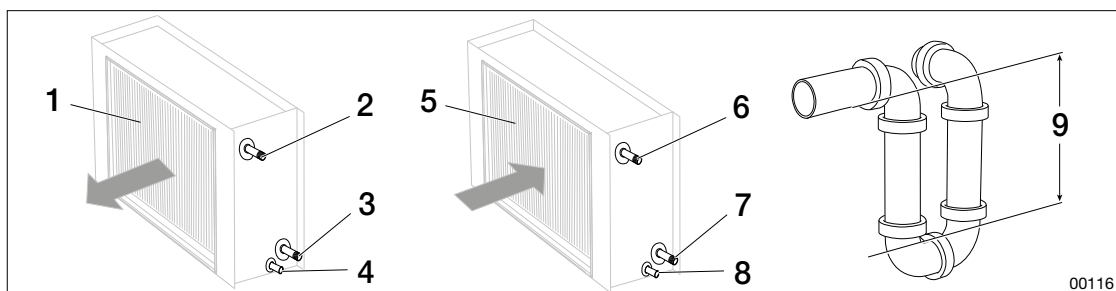
Ilustracja: Bateria chłodnicy (ETKB-VK)
