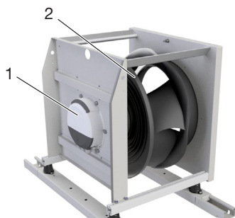
Eksempel på ventilator størrelse 240-1540
