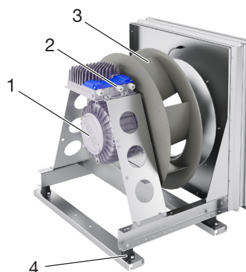
Eksempel på ventilator størrelse 480-1540
