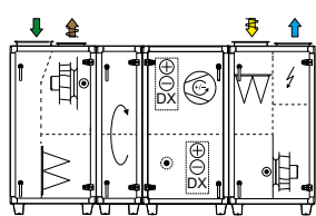
Rotor og køle-/varmepumpe størrelse 09, 12, 17 og 22
