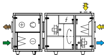
Med kølemaskine, tilluft nedad
