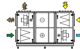
Komb. 11 Genvindingsbatteridel
