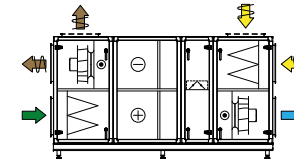
Komb. 13 Genvindingsbatteridel og recirkuleringsdel
