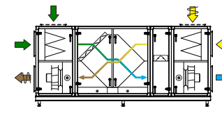
Komb. 9 Modstrømsveksler og recirkuleringsdel
