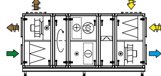
Komb. 5 Rotor, kølemaskine og recirkuleringsdel
