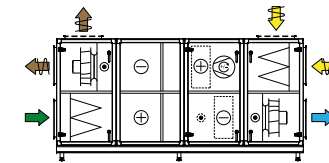
Komb. 12 Genvindingsbatteridel og kølemaskine
