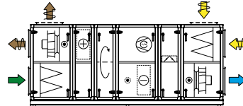
Komb. 6 Kølemaskine med kølegenvinding og recirkuleringsdel
