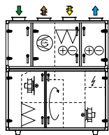
Rotor og køle-/varmepumpe størrelse 06 og 10
