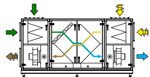
Komb. 7 Modstrømsveksler
