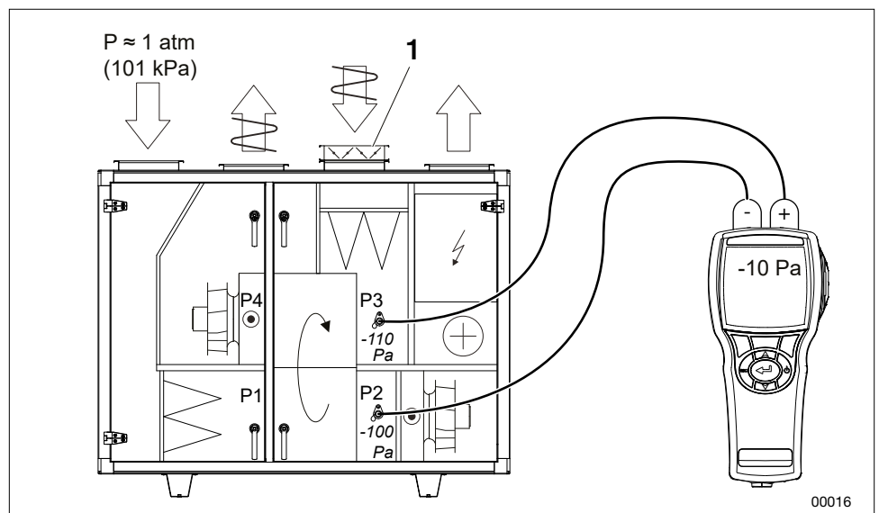
Måleuttak for trykktalanse – aggregat i utførelsen Home Concept.
