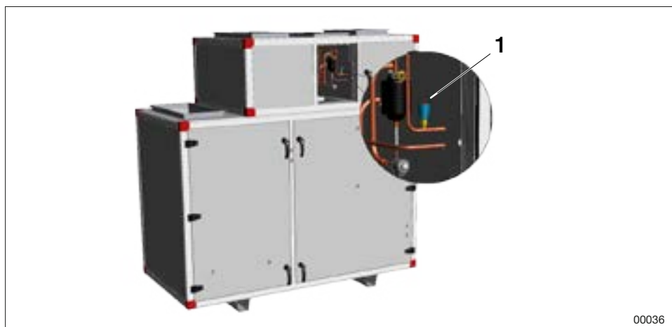
1. Tilbakestillingsknapp pressostat
