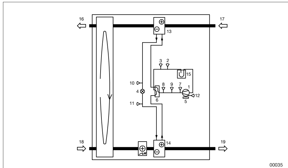
Systembilde for kjølemodus reversibel varmepumpe
