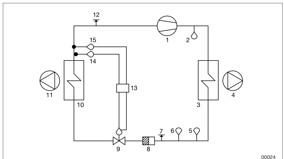
Flödesschema för köldmediesystem storlek 04-12
