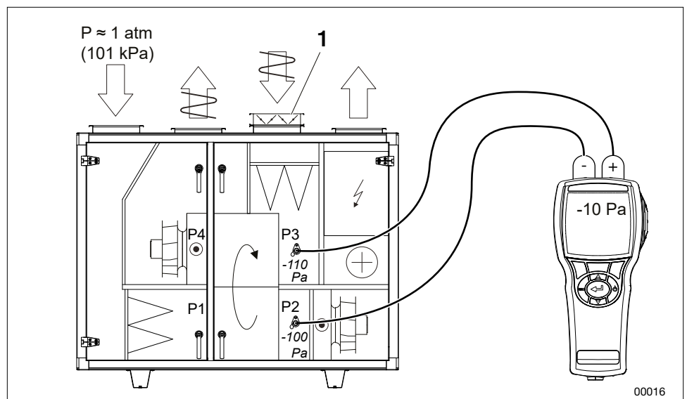
Mätuttag för tryckbalans - aggregat i utförande Home Concept
