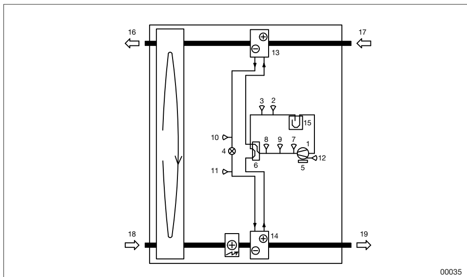
Flödesschema för kyl läge kylvärmepump
