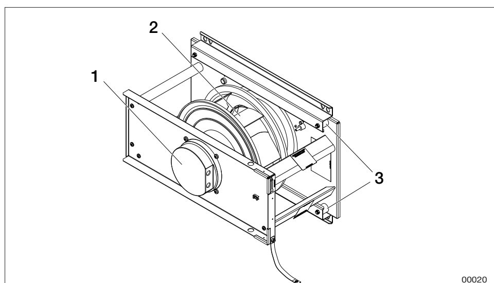
Exempel fläktenhet storlek 04-06
