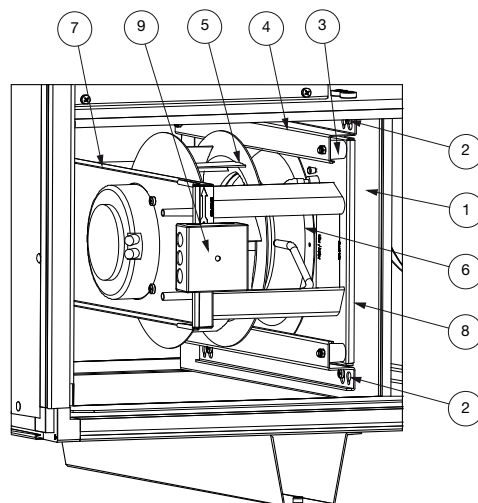
Fläktenhet storlek 04
