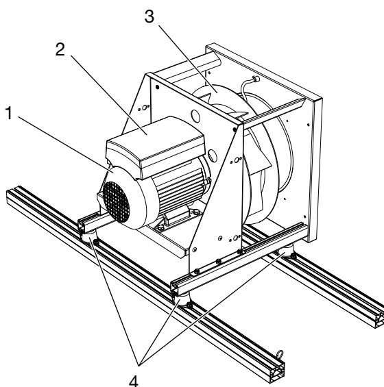
Fläktenhet
