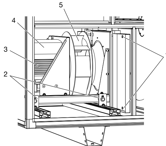
Fläktenhet storlek 06 och 10
