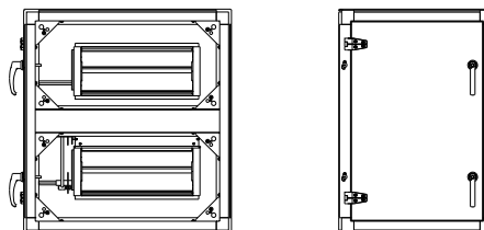
Внутренние оси (EBC-xxx-xx-I)
