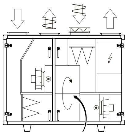
Återvinnare rotor
