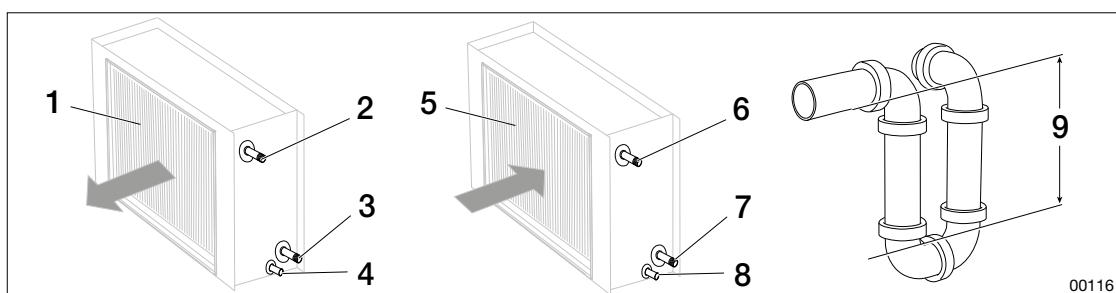
Figur: Kjølebatteri (ETKB-VK)
