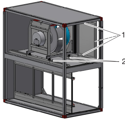
Voorbeeld ventilatoreenheid
