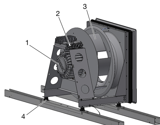
Ventilatoreenheid grootte 480-1540
