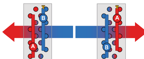
Abbildung: Anschluss Rohr, Heizregister (ECET-VV)
