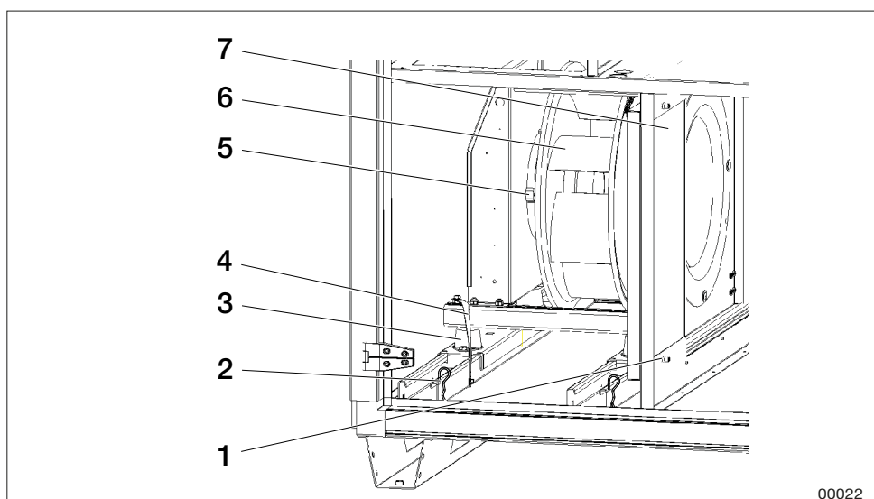
Voorbeeld ventilator grootte 09-28
