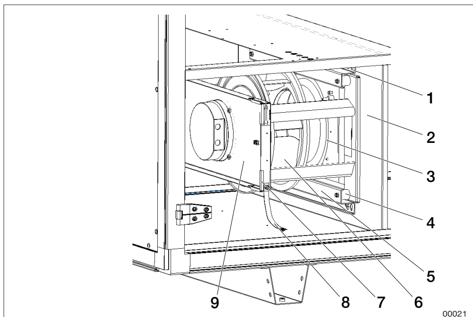
Voorbeeld ventilatoreenheid grootte 04-06 met ventilatorwiel 025
