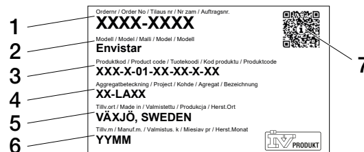
Voorbeeld Typeplaatje unit
