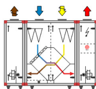
Delt utførelse størrelse 04, 06 og 10
