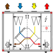
Enhetsutførelse størrelse 04, 06 og 10
